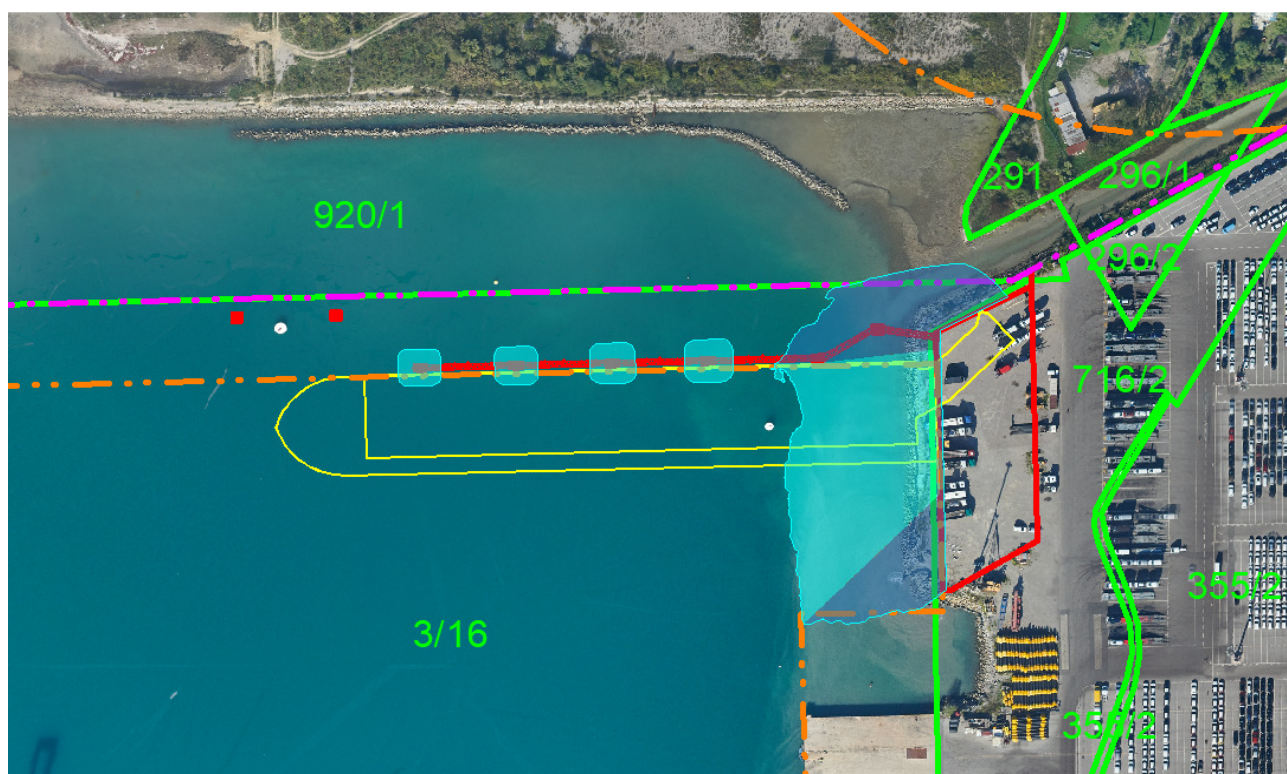
SLIKA 3: PRIKAZ LOKACIJE POSEGA PRIVEZ (OBMOČJE KONSTRUKCIJE - RDEČA BARVA, OBMOČJE IZKOPA NA -10M Z BREŽINO - SVETLO MODRA BARVA, MEJE PARCEL - ZELENA BARVA, MEJA OBMOČJA KOPRSKEGA TOVORNEGA PRISTANIŠČA V SKLADU Z UREDBO O UPRAVLJANJU KOPRSKEGA TOVORNEGA PRISTANIŠČA – ROZA BARVA, MEJA KOPENSKEGA DELA OBMOČJA PRISTANIŠČA V SKLADU Z DRŽAVNIM PROSTORSKIM NAČRTOM – ORANŽNA BARVA)
