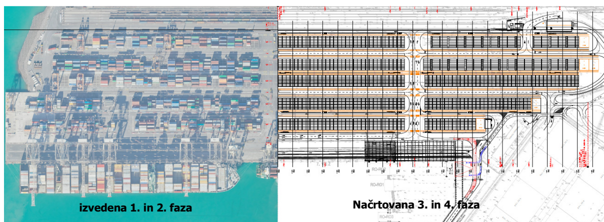
Slika 2: Pomol I - ortofoto območja ureditve kontejnerskega terminala 1. in 2. faze ter prikaz projektiranega stanja 3. in 4. faze (interni vir)
