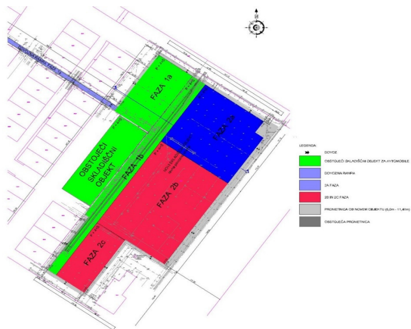
Slika 1: Prikazan je »NOV SKLADIŠČNI OBJEKT ZA AVTOMOBILE V LUKI KOPER«. Z zeleno šrafuro so označene že zgrajene faze. Z modrim je označena FAZA 2A, ki je predmet tega naročila. Z rdečo so prikazane bodoče faze, ki niso predmet tega naročila.
