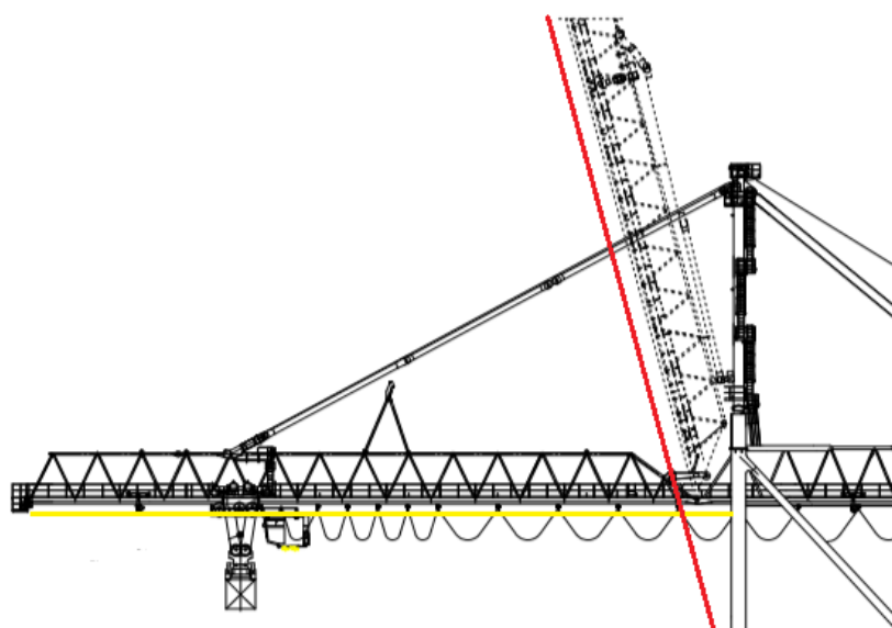
Slika 1: Območje varovanja roke
