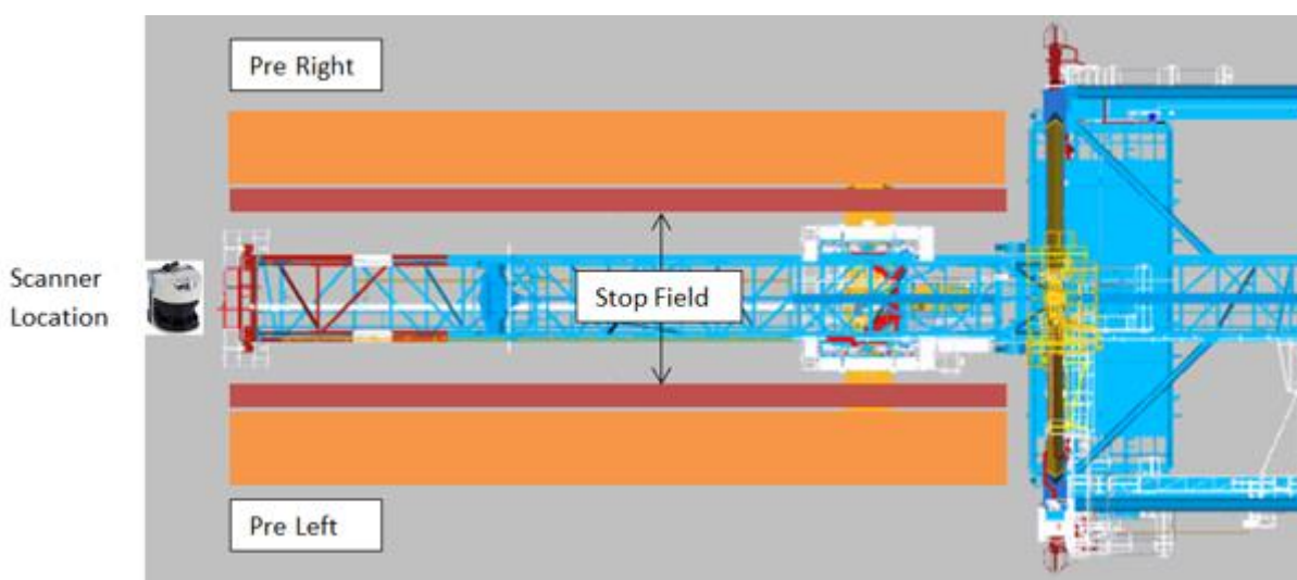
Slika 2: Prikaz lokacije montaže senzorja, prikaz pred izklopa ter prikaz končnega izklopa vožnje dvigala
