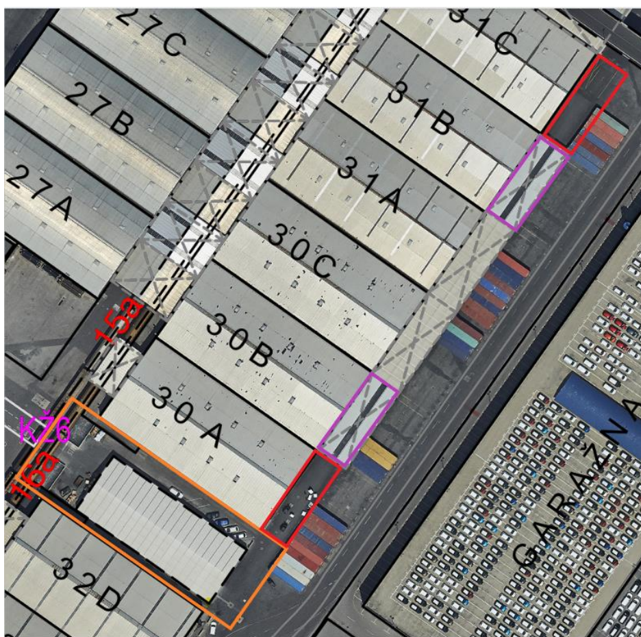
Slika: lokacija posega (oranžna barva (sklop 1): območje bodočega skladišča 32E in nadstrešnice, vijola in rdeča barva (sklop 2): območje nadstrešnic pred obstoječimi skladišči)
