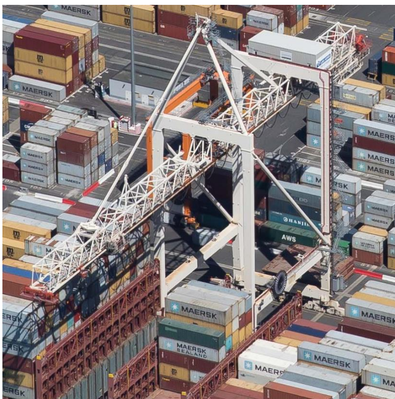
Slika 1: Kontejnersko dvigalo KD 56 (IR1773)
