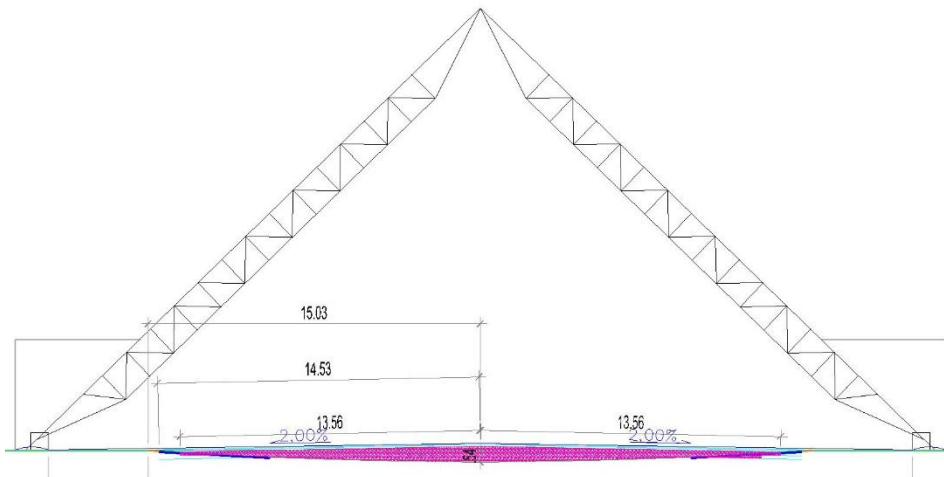
Slika 3. Tehnična rešitev za izvedbo sanacije –prečni prerez TH 1 hale.
