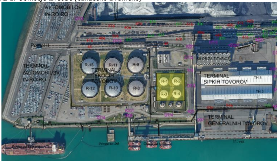
Slika 2: Rezervoarji za plinsko in lahko kurilno olje
