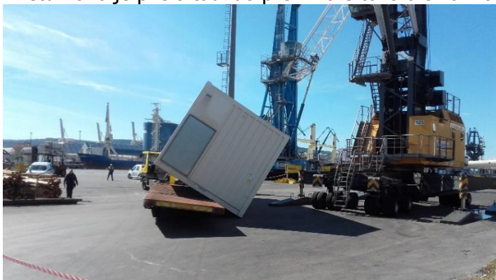
Slika 1: Prevrtitev tovora kot posledica neustreznih naklonov
