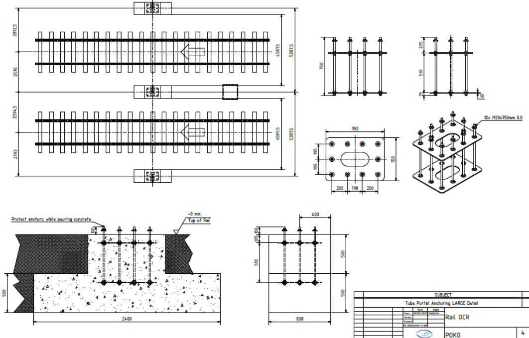
Slika 4. Načrt temeljev
