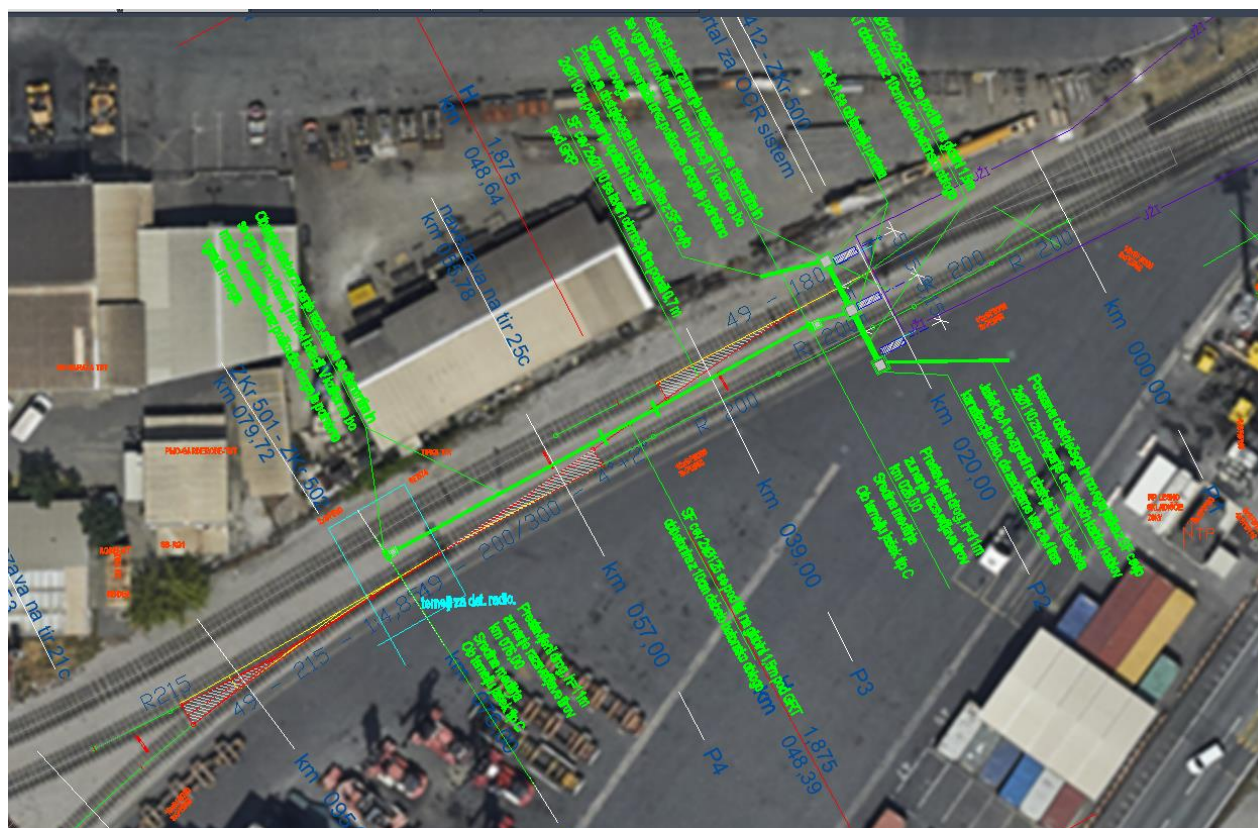
Slika 2. Prikaz lokacije temeljev in elektrokabelske kanalizacije s priklopi
