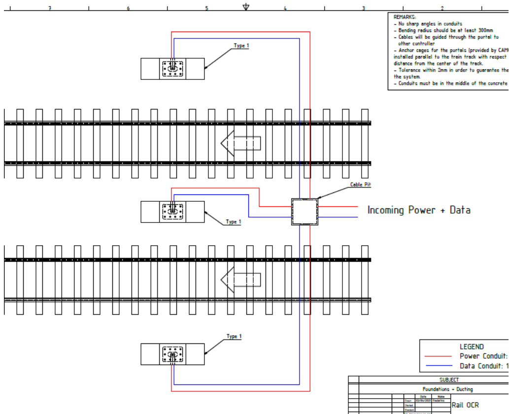
Slika 5. Shematski prikaz elektrokabelske in TK kanalizacije
