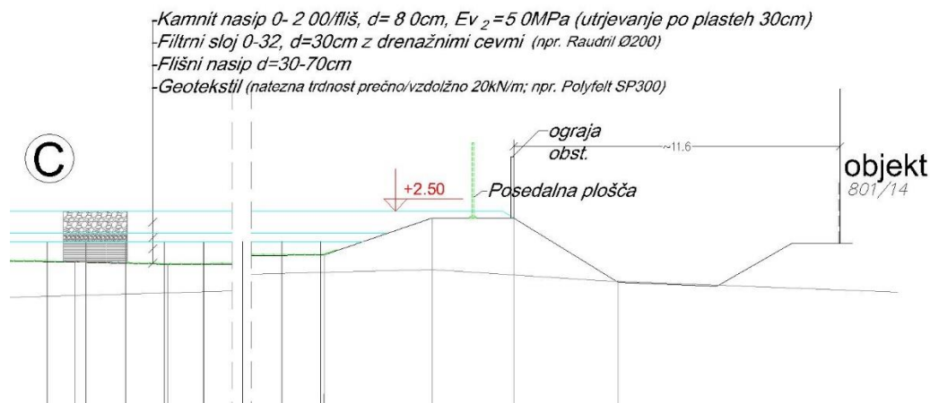
SLIKA 2: KARAKTERISTIČNI PREREZ PREDOBREMENILNEGA NASIPA
