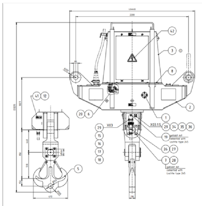
Slika 3: Primer kavlja dvigala Liebherr LHM 150 in Fantuzzi MHC 115
