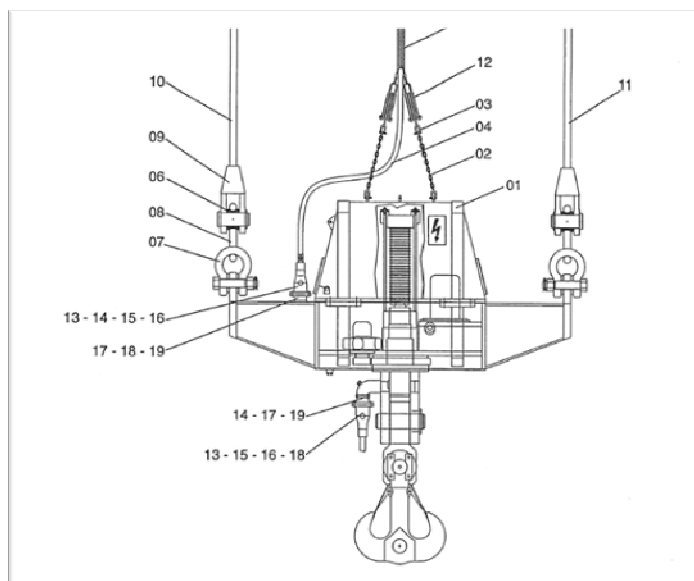
Slika 3: Primer kavlja dvigala Liebherr LHM 150 in Fantuzzi MHC 115
