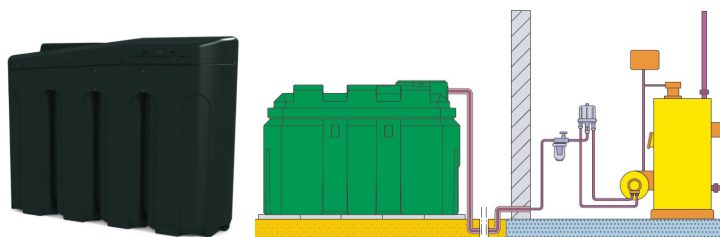
Slika 4: Primer nadzemnega rezervoarja iz umetne mase ter primer postavitve
